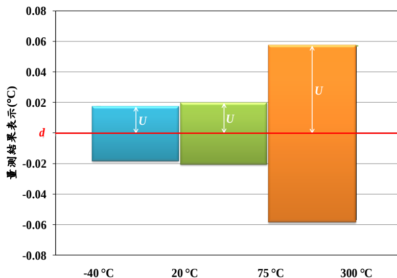
電阻溫度計之最小擴充不確定度
