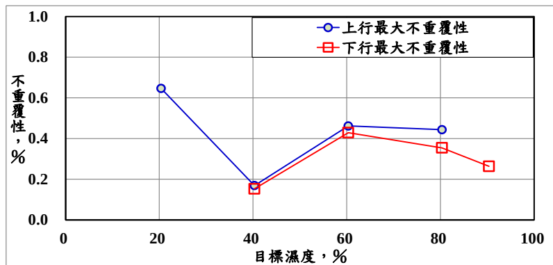
產品不重複性曲線
