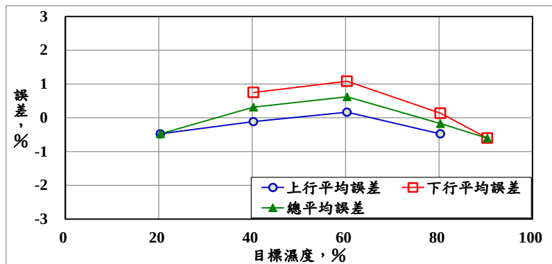
產品誤差曲線
