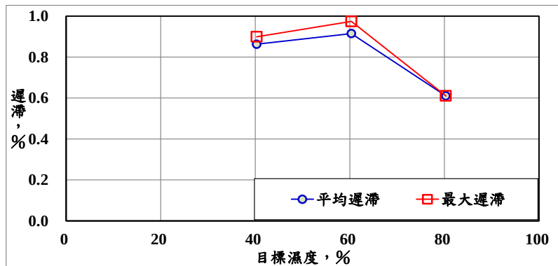
產品遲滯曲線
