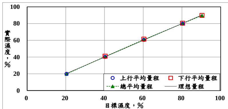
產品量程曲線
