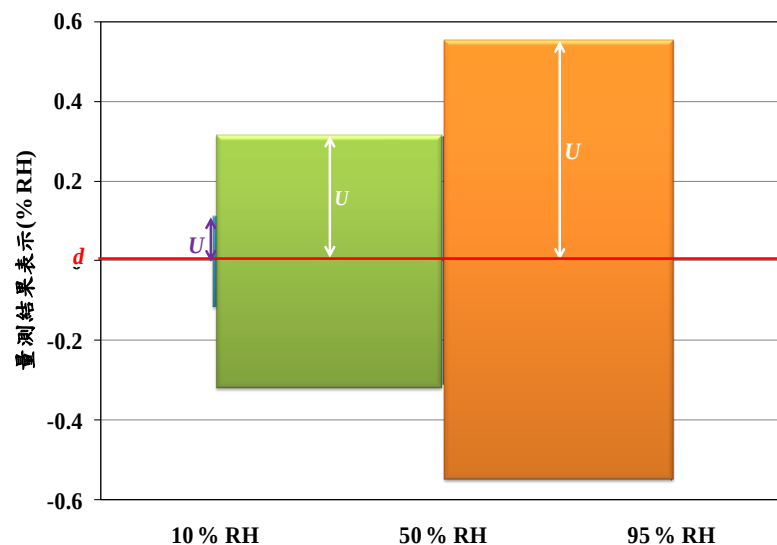
濕度計之最小擴充不確定度
