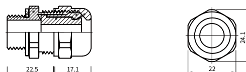
【N型(M16 金屬電纜固定座)】
